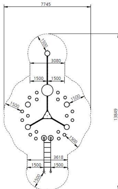
Wymiary strefy bezpieczeństwa
